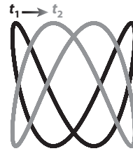
e Lissajous figure
